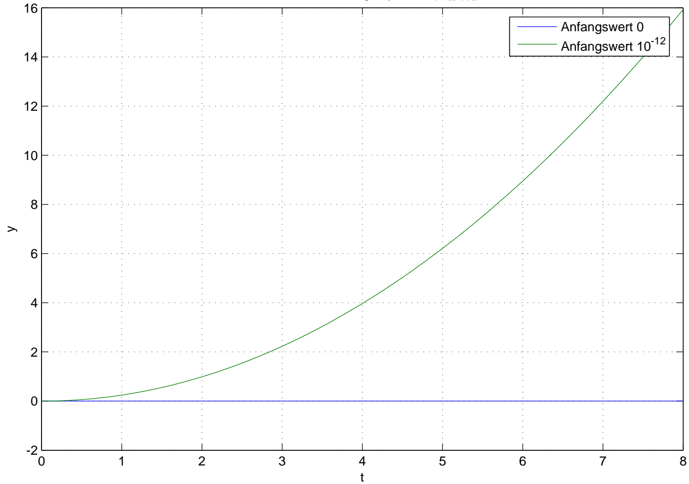
Die Instabilität der Dgl. dy/dt = \sqrt{|y(t)|}
