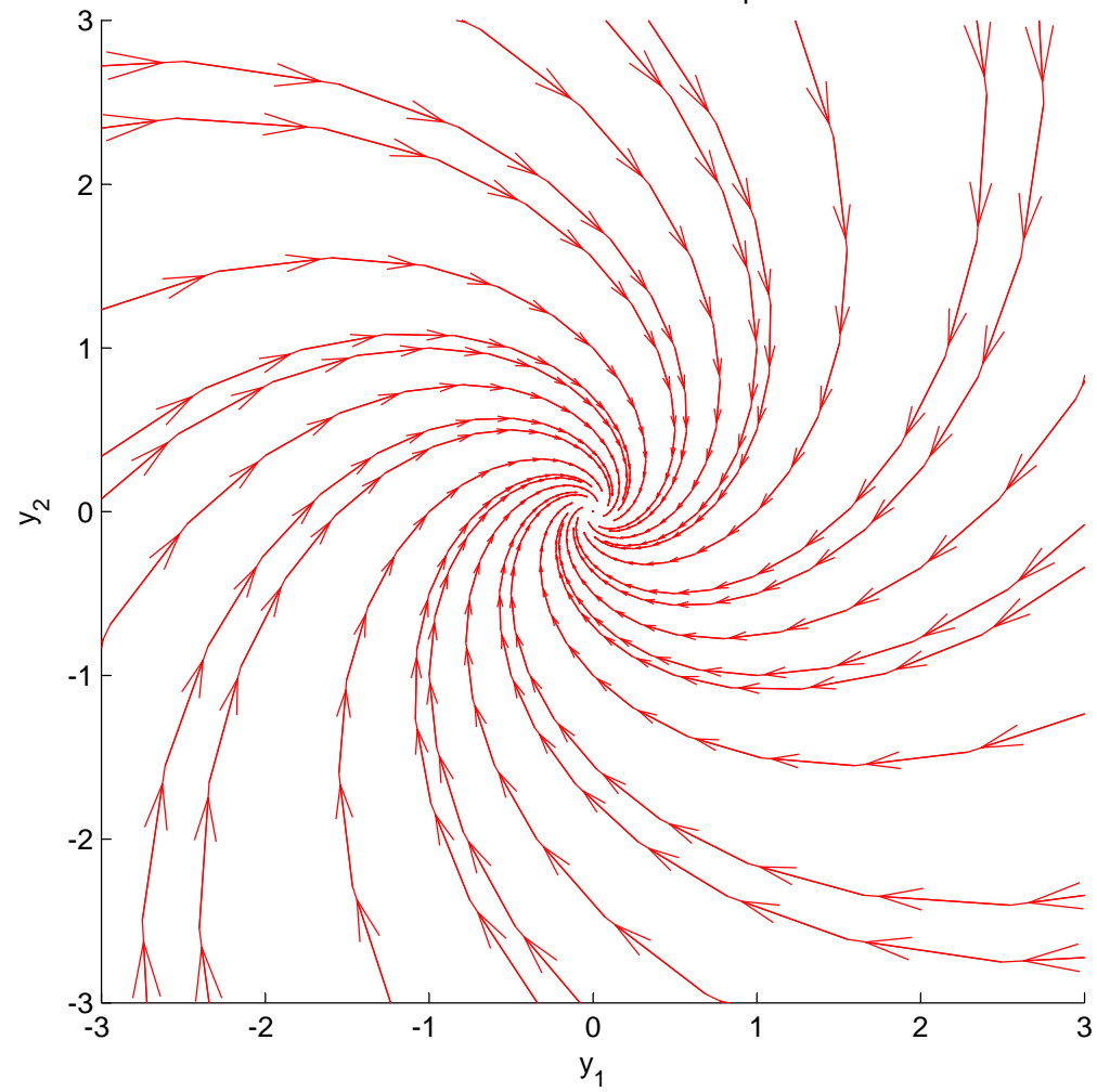
Zur Stabilität: stabiler Strudelpunkt
