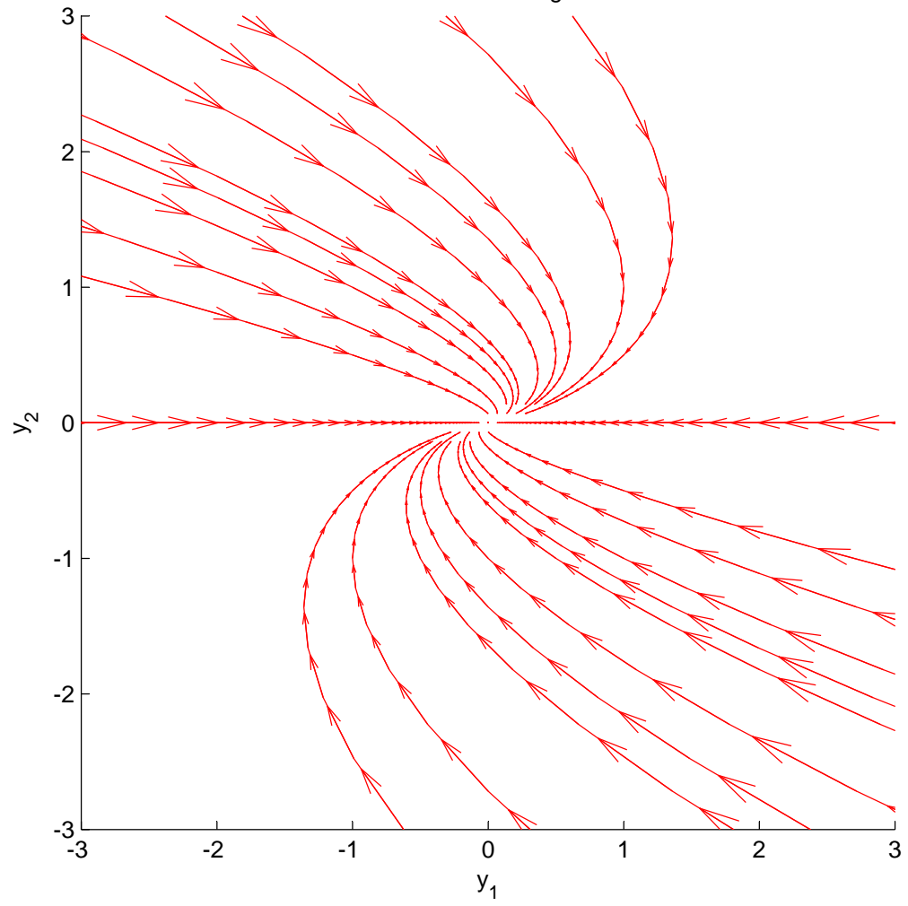
Zur Stabilität: stabiler eintangentialer Knoten
